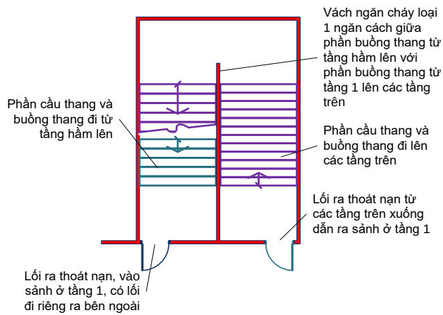
b) Mặt bằng
