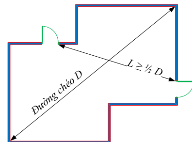
c) Xác định khoảng phân tán của các lối ra thoát nạn trong một số trường hợp mặt bằng phức tạp
